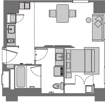
■ type B : 44m 2 /Queen
