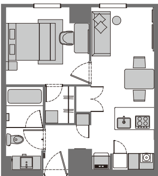
■ type C : 44m 2 /Queen
